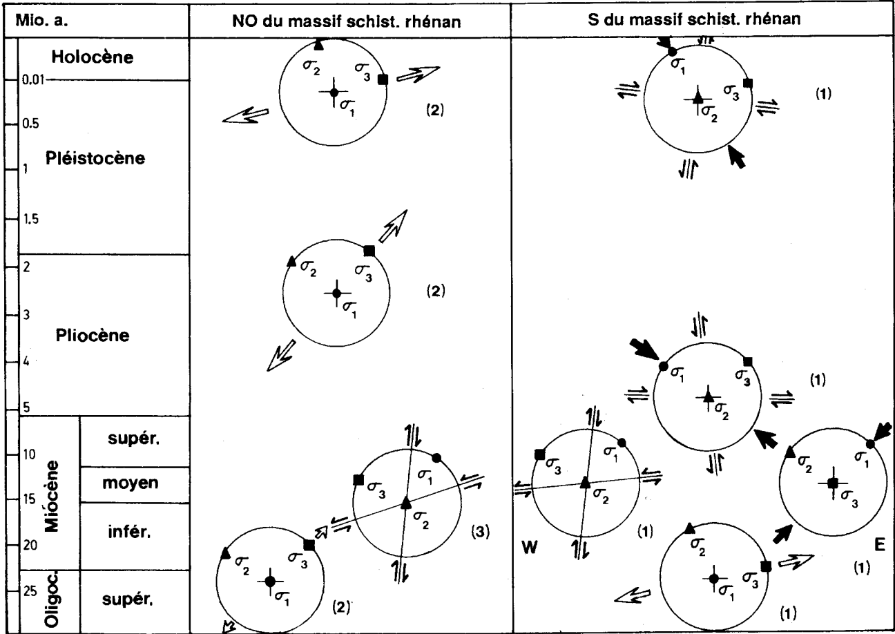
Fig. 5.- Directions des axes des contraintes principales en Europe occidentale depuis l'Oligocène supérieur.
