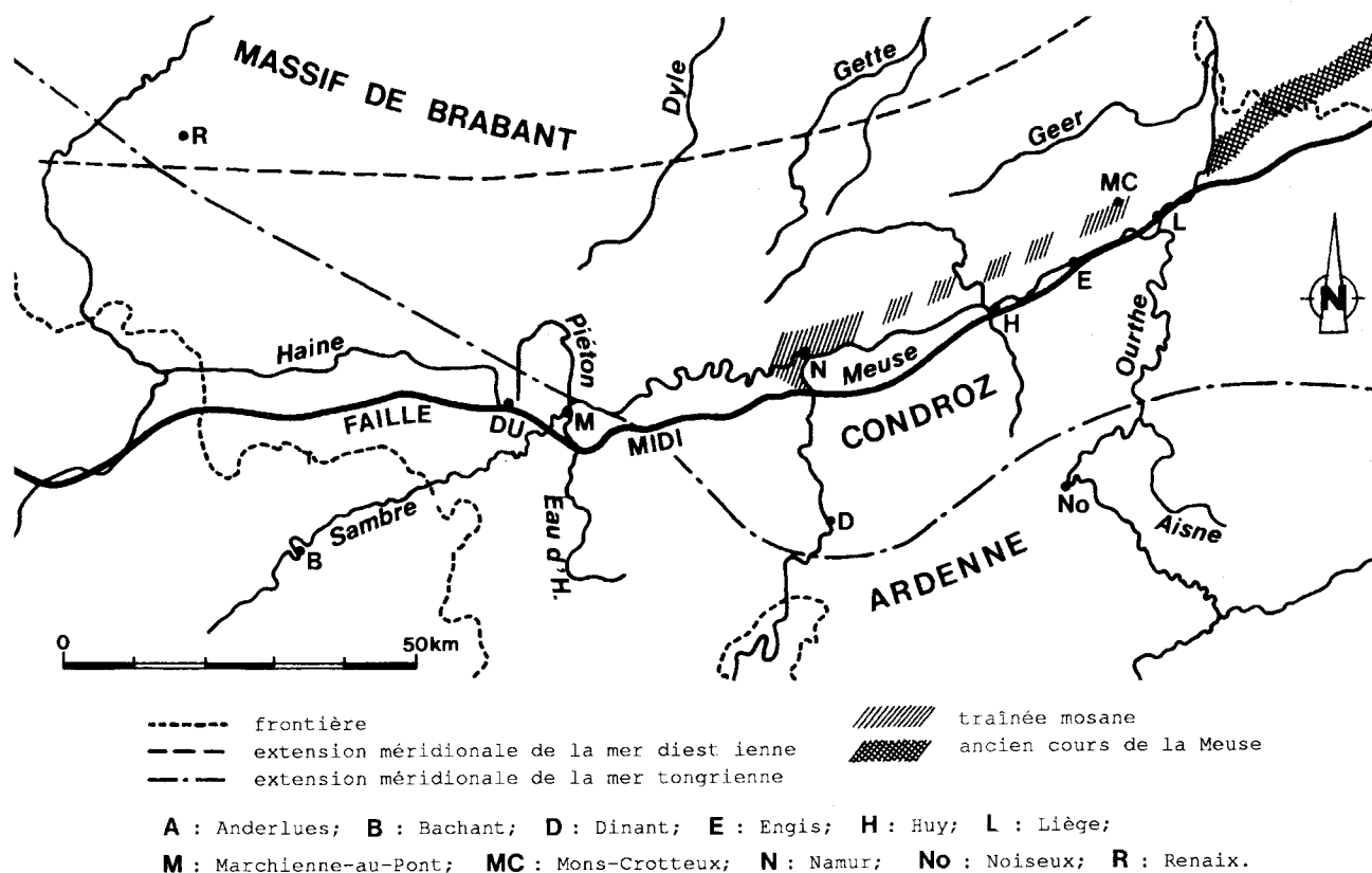
Fig. 1.- Situation du sillon sambro-mosan et limites méridionales des mers tongrienne et diestienne.
