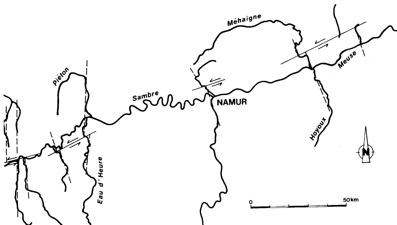
Fig. 6.- Décrochements senestres suggérés par des décalages dans le cours des affluents de la Sambre et de la Meuse.
