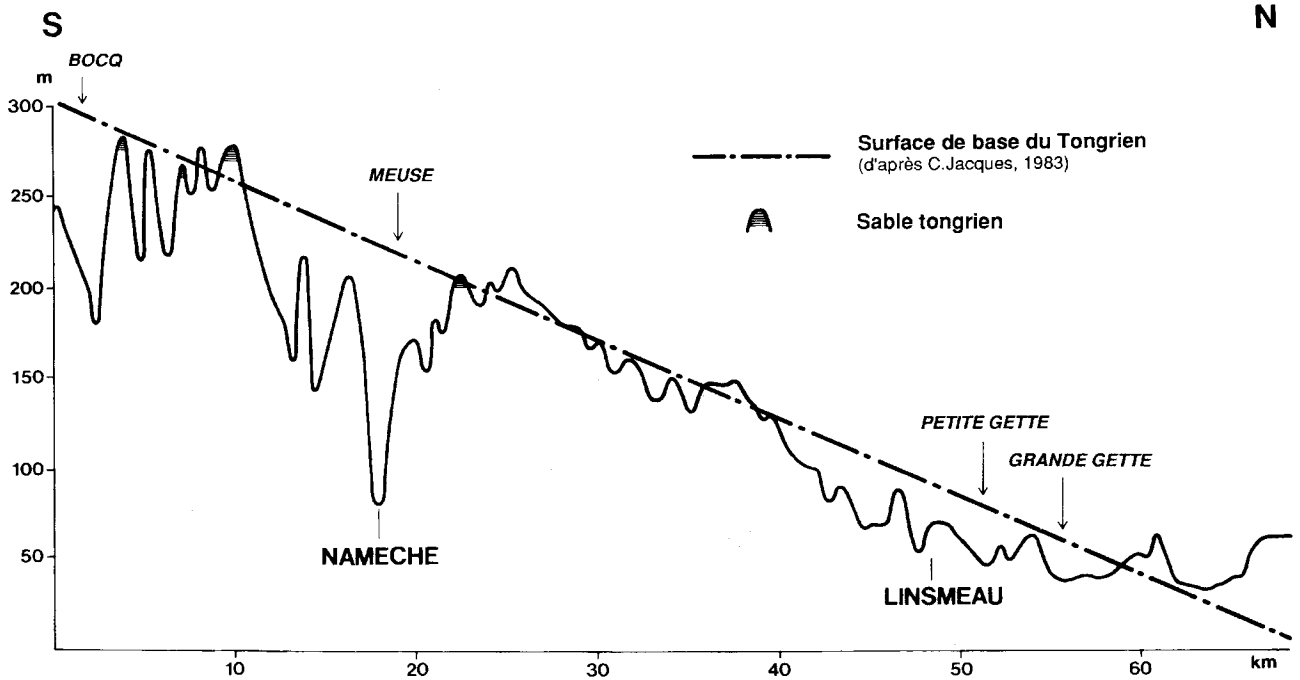
Fig. 4.- Profil topographique N-S recoupant la vallée de la Meuse à la hauteur de Namèche, et indiquant l'absence de déformations de la surface de base du Tongrien au passage du sillon mosan.
