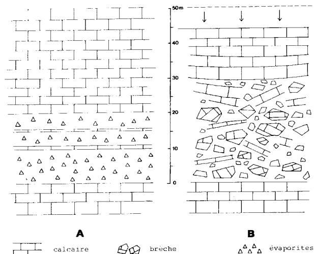
Fig. 3.- Développement de brèches d'effondrement suite à la dissolution d'évaporites.
