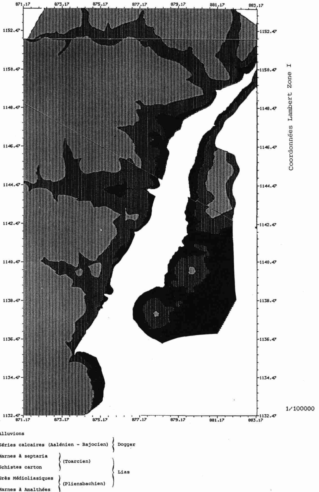
Figure 4.6. - Carte géologique
