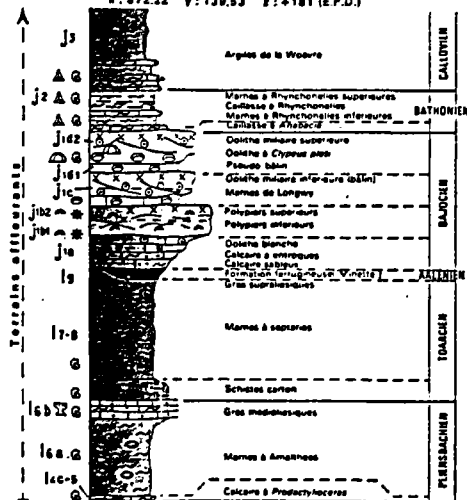
COUPE LITHOSTRATIGRAPHIQUE établie d'après les terrains affleurants et le forage de Pont-à-Mousson n° 4-3 N : 872.22 V : 139.53 Z : +181 (E.P.D.)
