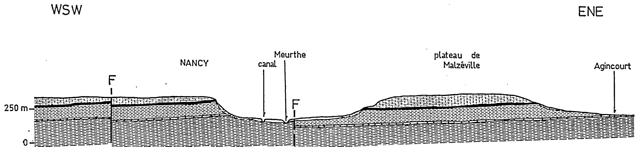
FIG.2.1 - Coupe géologique synthétique interprétative
