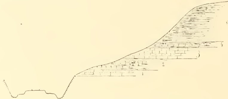
FIG. 2. — Coupe de la tranchée du chemin de fer de Villers-sur-Semois.
