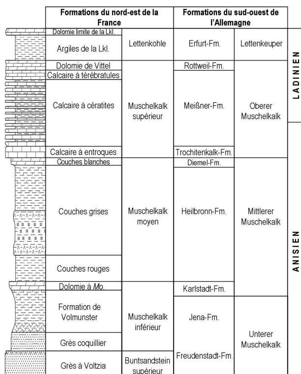
Figure 2 – Série lithostratigraphique du Trias moyen de Lorraine comparée à celle du sud-ouest de l'Allemagne d'après Durand & Hagdorn (2021). Lkl. : Lettenkohle ; Mo. : Myophoria orbicularis ; Fm. : Formation.
