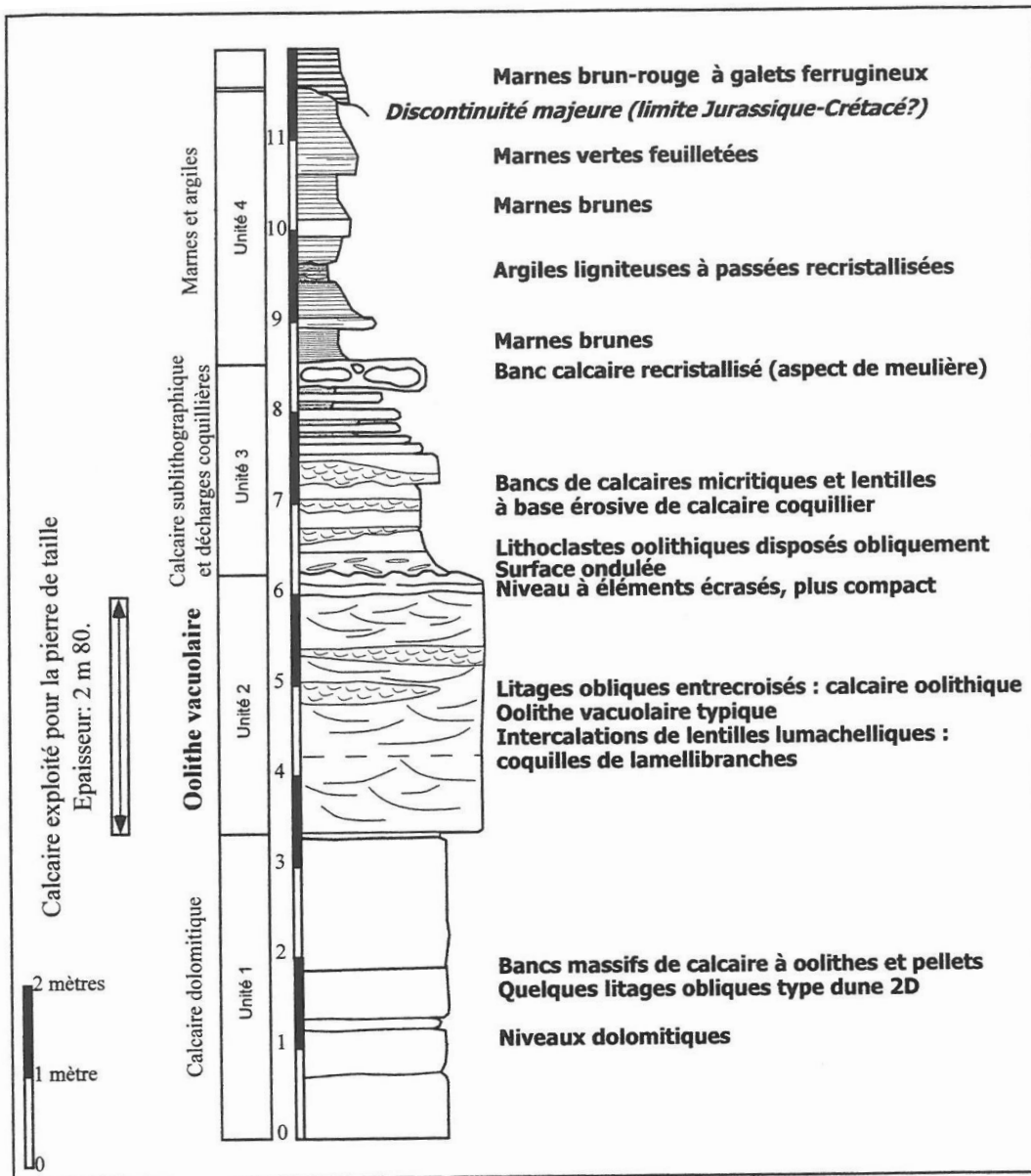
Fig. 2 : Log de la carrière de la Fontaine, Brauvilliers (55) Oolithe vacuolaire, calcaires et marnes de la fin du Tithonien
