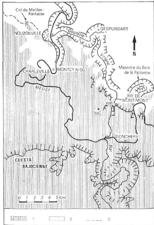
FIGURE 3. Tracé actuel de la Meuse à la bordure sud de l'Ardenne. Sur cette figure apparaît la vallée morte passant par Gespunsart (où coulent la Goutelle et la Vrine) que la Meuse empruntait avant d'être détournée vers Charleville par la Bar. Au nord-ouest de cette figure est dessiné en tiretés le tracé probable de la Meuse avant la capture de la Meuse lorraine par la Meuse de Dinant qui passait par le col de Meillier-Fontaine.
