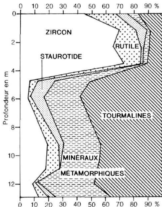
FIGURE 10. Les minéraux lourds de la sablière d'Opgimbe au nord de Maastricht.
