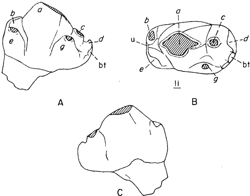
Fig. 7. Brachyzostrodon coupatezi gen.n., sp.n., SNP 68 W; molaire inférieure droite, A vue linguale; B vue occlusale; C vue labiale; \times 20 . ll côté lingual; bt, cr, u, uc voir texte.
