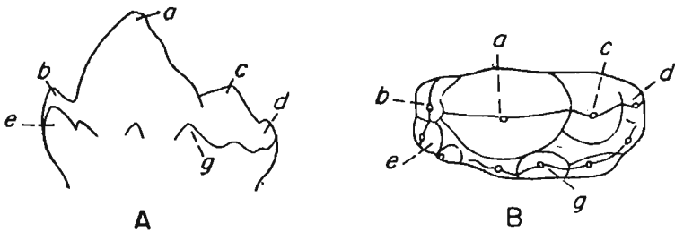
Fig. 8. Brachyostrodon coupatezi gen.n., sp.n., SNP 108 W; molaire inférieure droite. A vue linguale; B vue occlusale; X20.
