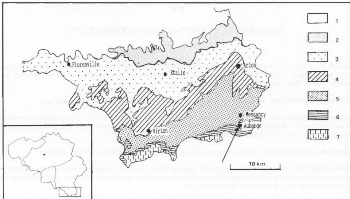
Figure 1. Cadre géologique régional et localisation géographique des environs d'Aubange (Fleche). 1: socle ardennais; 2: Trias supérieur; 3: Hettangien et Sinemurien inférieur; 4: Sinemurien supérieur; 5: Pliensbachien; 6: Toarcien; 7: Bajocien.
