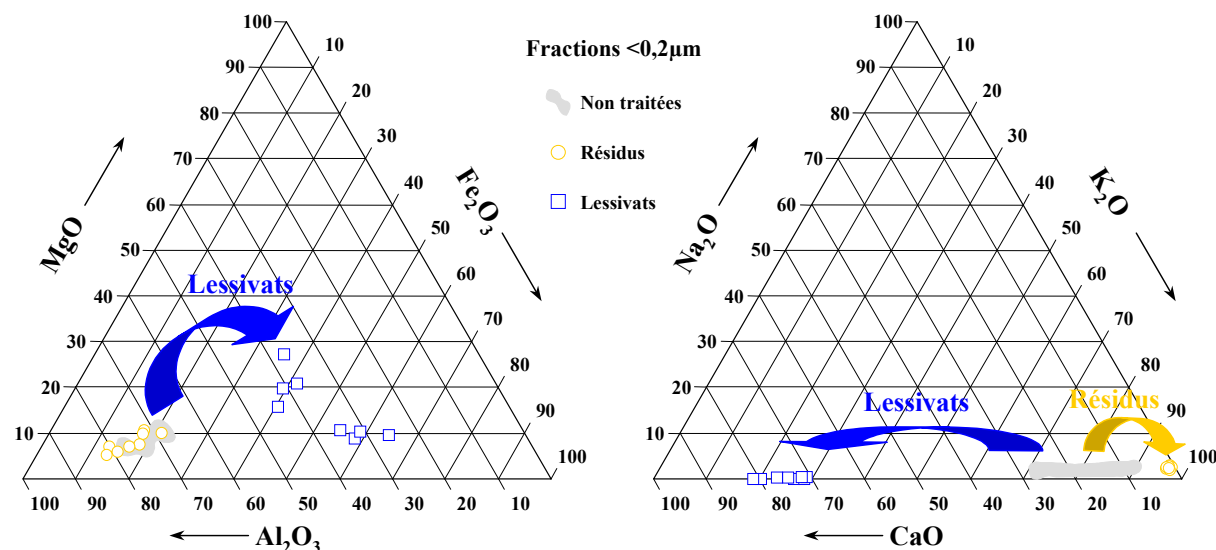
Figure IV-23 : Compositions chimiques des fractions <0,2µm reportées dans un diagramme Al_2O_3 - Fe_2O_3 - MgO (à gauche) et un diagramme CaO - Na_2O - K_2O (à droite) avant (domaine grisé) et après lavage HCl (Résidus et lessivats).
