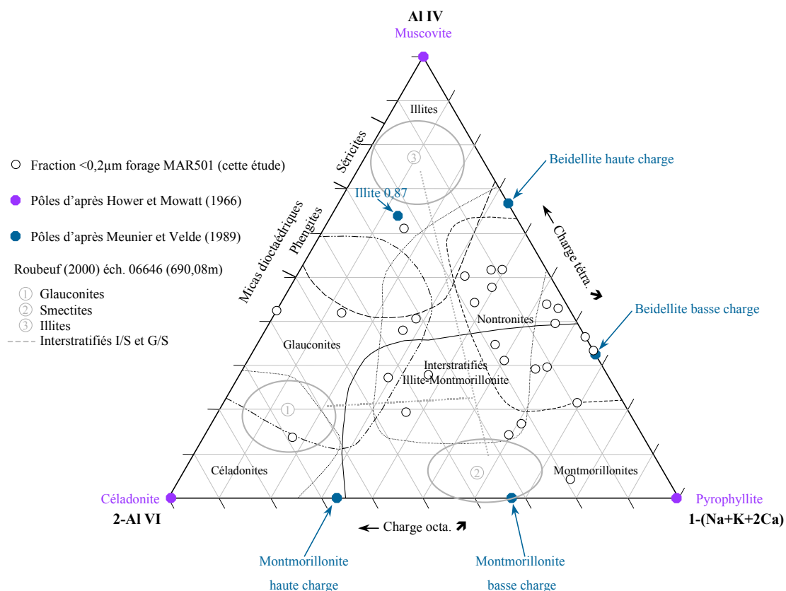
Figure VI-3 : Diagramme CMP de la fraction <0,2µm (forage MAR501). Les domaines de répartition des charges (en équivalents pour 22 valences négatives) dans les formules structurales d'illites, de glauconites, de céladonites, d'interstratifiés illite/montmorillonite et de smectites sont extraits de Duplay (1982) d'après Weaver et Pollard (1973).
