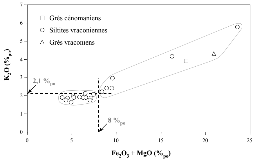
Figure VI-5 : Corrélations entre les teneurs en Fe_2O_3+MgO et les teneurs en K_2O dans la fraction <2\mu m (forage MAR501).
