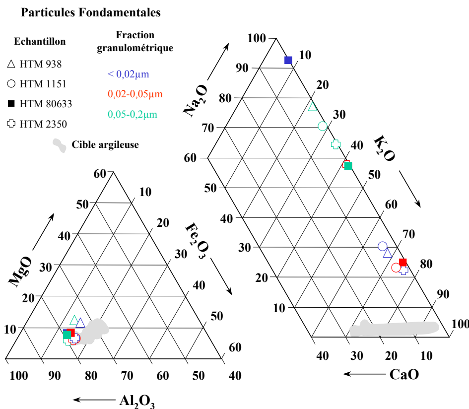
Figure IV-13 : Compositions chimiques des particules fondamentales reportées dans un diagramme Al_2O_3 - Fe_2O_3 - MgO (à gauche) et un diagramme CaO - Na_2O - K_2O (à droite). Les symboles distinguent chaque échantillon et les couleurs chaque fraction granulométrique (domaine grisé : cible argileuse, figures IV-7&8).
