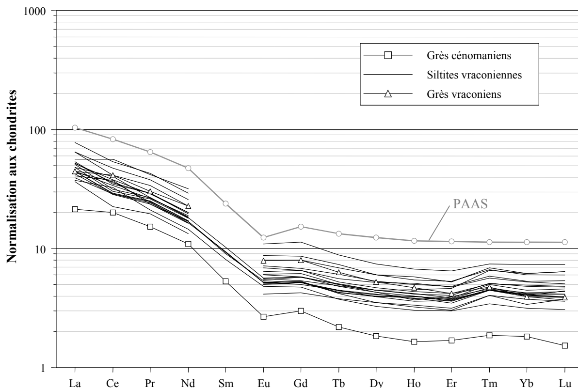
Figure VI-8 : Spectres de terres rares normalisés par rapport aux chondrites de la fraction <2µm (forage MAR501). Le spectre correspondant aux PAAS a également été reporté pour comparaison. Les spectres sont similaires bien que les argiles de la séquence du Gard présentent des teneurs plus faibles que celles des PAAS. Les grès cénomaniens sont caractérisés par les teneurs en terres rares les plus faibles.
