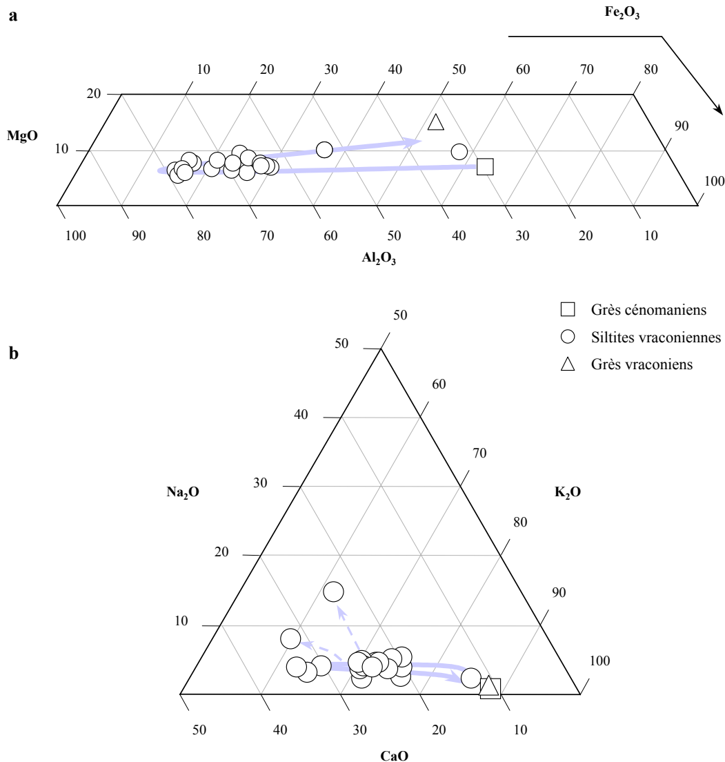
Figure VI-4 : Diagrammes triangulaires Al_2O_3 - Fe_2O_3 - MgO (a) et CaO - Na_2O - K_2O (b) de la fraction <2\mu m (forage MAR501).
